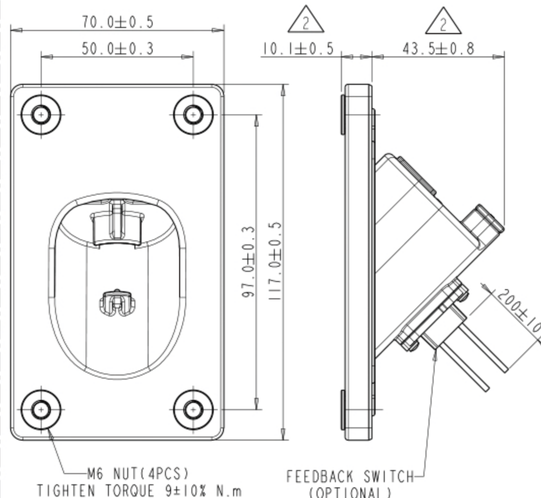
NUT TYPE
